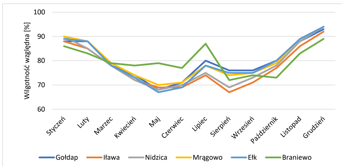
Rysunek 1-20 Przebiegi średnich miesięcznych wartości wilgotności powietrza wyznaczone przez model WRF/CALMET w wybranych miejscowościach strefy warmińsko-mazurskiej w 2018 r.
