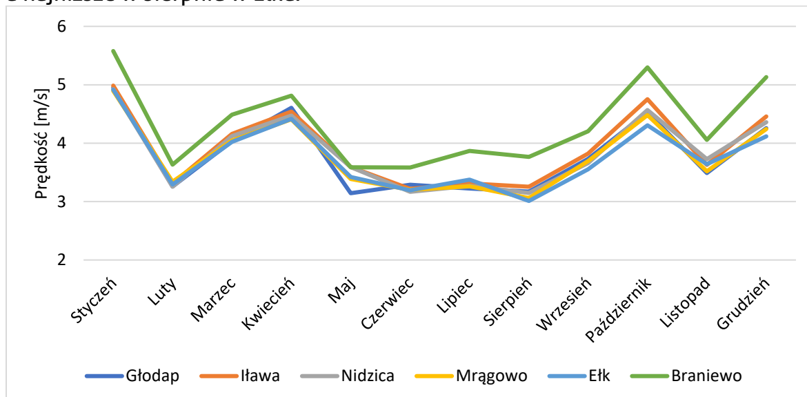
Rysunek 1-8 Średnia miesięczna prędkość wiatru wyznaczona przez model WRF/CALMET dla wybranych miejscowości w strefie warmińsko-mazurskiej w 2018 r.
