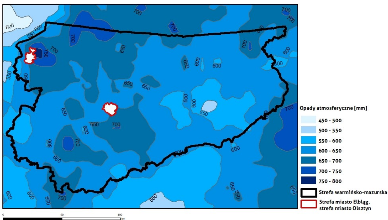
Rysunek 1-17 Przestrzenny rozkład rocznych sum opadów atmosferycznych wyznaczonych przez model WRF/CALMET w strefie warmińsko-mazurskiej w 2018 r.
