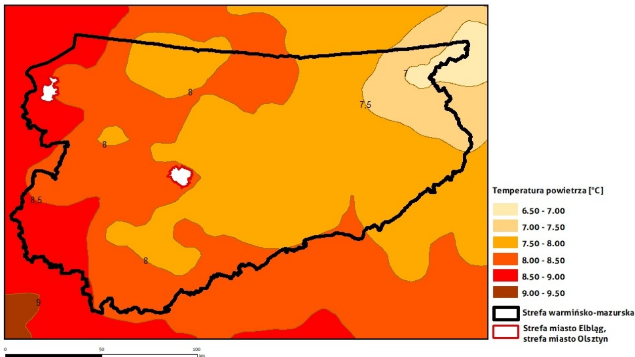
Rysunek 1-14 Przestrzenny rozkład średnich rocznych wartości temperatury powietrza wyznaczonych przez WRF/CALMET w strefie warmińsko-mazurskiej w 2018 r.
