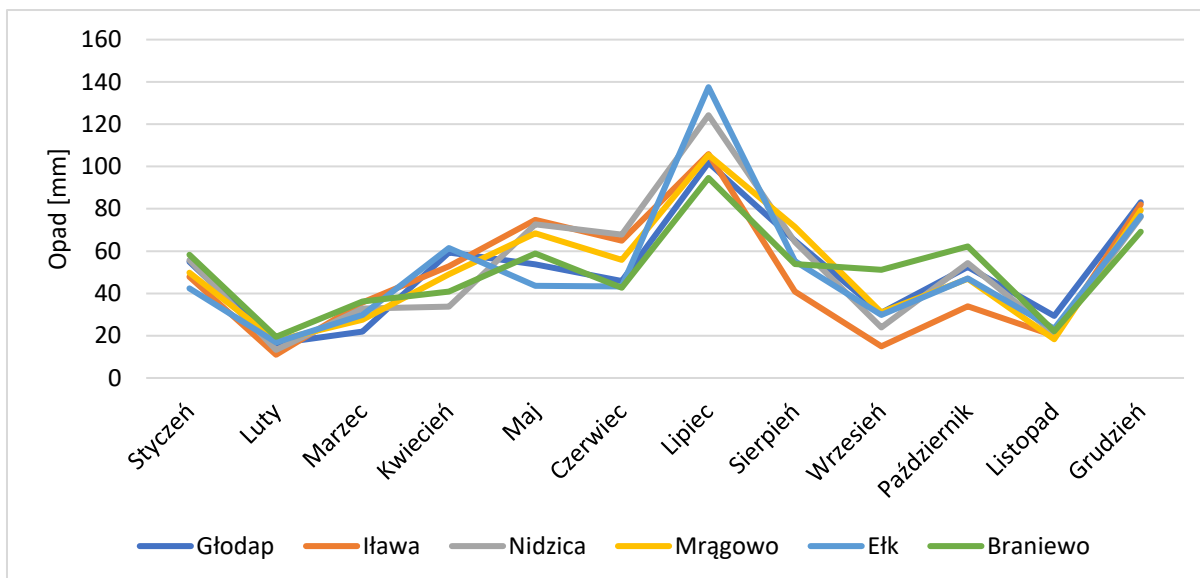
Rysunek 1-18 Miesięczne sumy opadów atmosferycznych wyznaczone przez modele WRF/CALMET w wybranych miejscowościach strefy warmińsko-mazurskiej w 2018 r.
