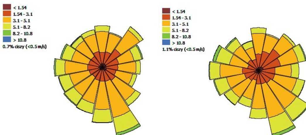
Rysunek 1-13 Rozkład kierunków i prędkości wiatru odpowiednio dla Mrągorowa i Nidzicy w 2018 r.
