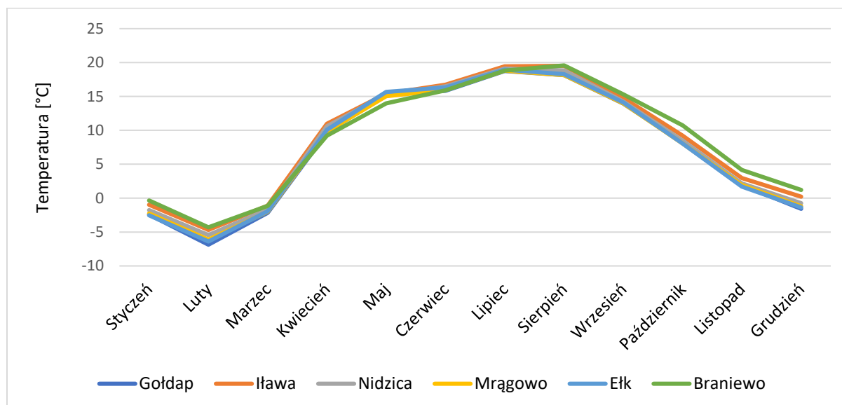
Rysunek 1-15 Przebiegi średnich miesięcznych temperatur powietrza wyznaczone przez model WRF/CALMET w wybranych miejscowościach strefy warmińsko-mazurskiej w 2018 r.
