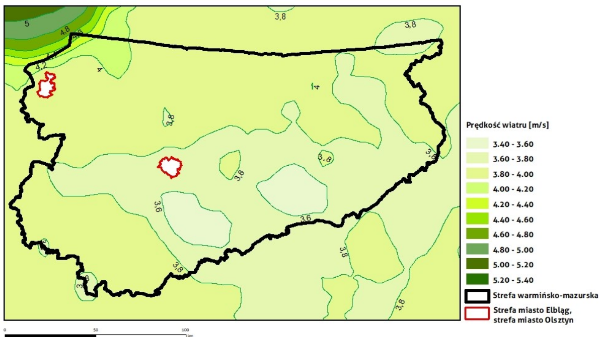
Rysunek 1-6 Przestrzenny rozkład średnich rocznych prędkości wiatru wyznaczonych przez model WRF/CALMET w strefie warmińsko-mazurskiej w 2018 r.
